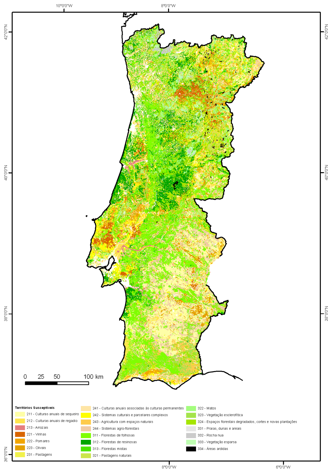
Figura 5 – Territórios suscetíveis a incêndios florestais (Fonte: Corine Land Cover 2000)
