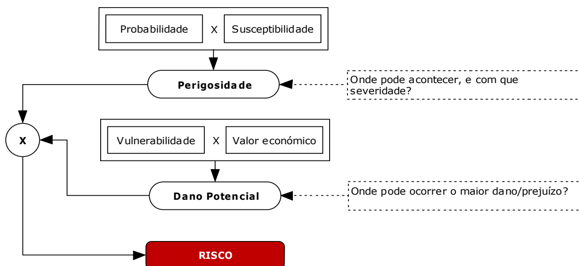
Figura 3 – Componentes do modelo de risco
